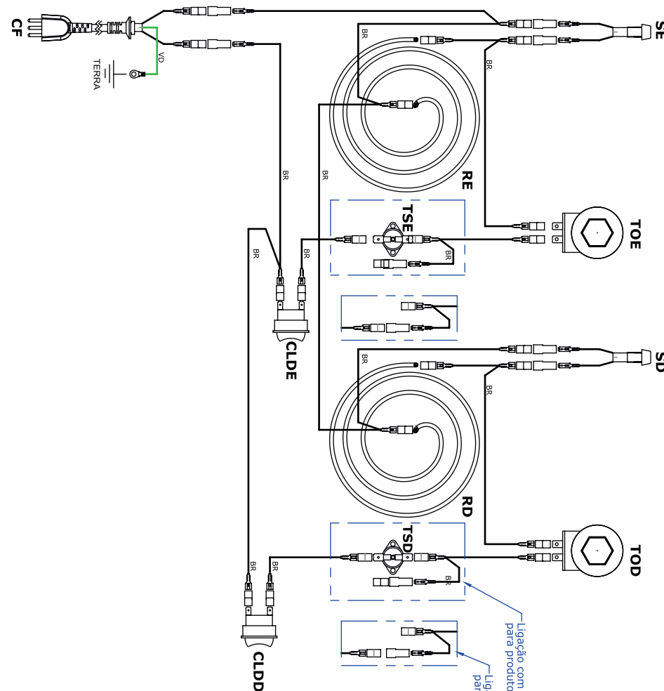
Diagrama Elétrico PRKF-202 E Style (127V ou 220V) DEP25:
